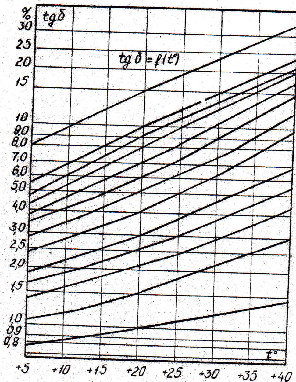
Рис. 2 Зависимость угла диэлектрических потерь от температуры для бакелитовых бумажных вводов.
