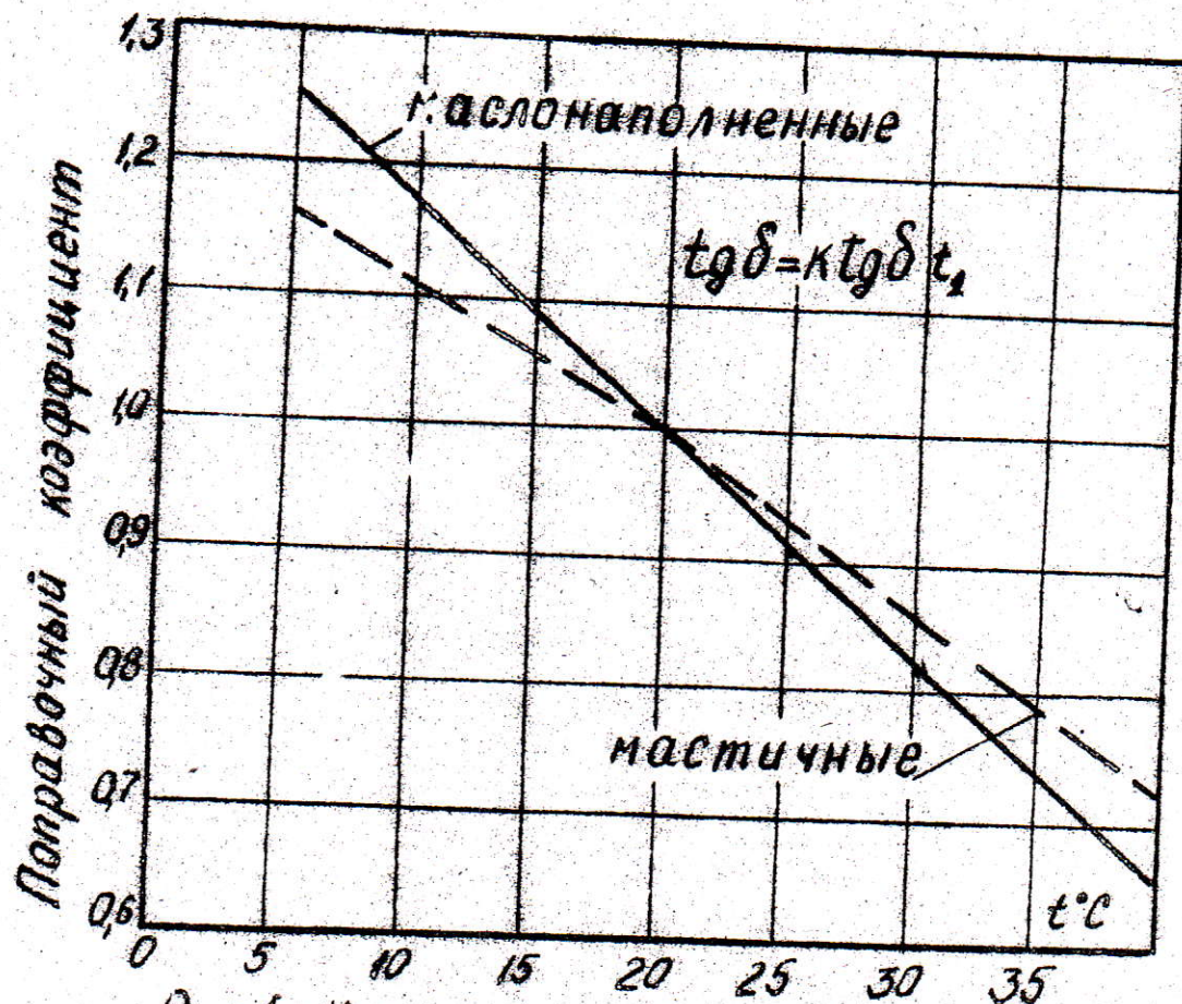
Рис. 1 Кривые поправочных коэффициентов \text{tg}\delta на температуру для маслонаполненных и мастичных вводов и ТН.
